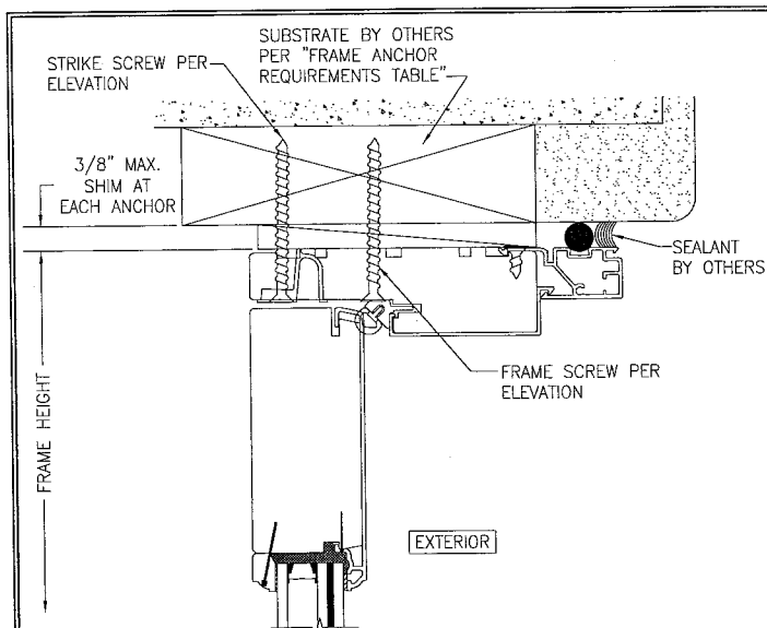
SECTION A3 SCALE: 1/2 FULL
